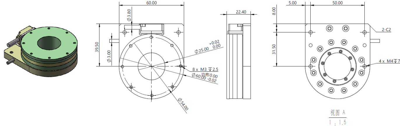
ACR60-022安装尺寸
