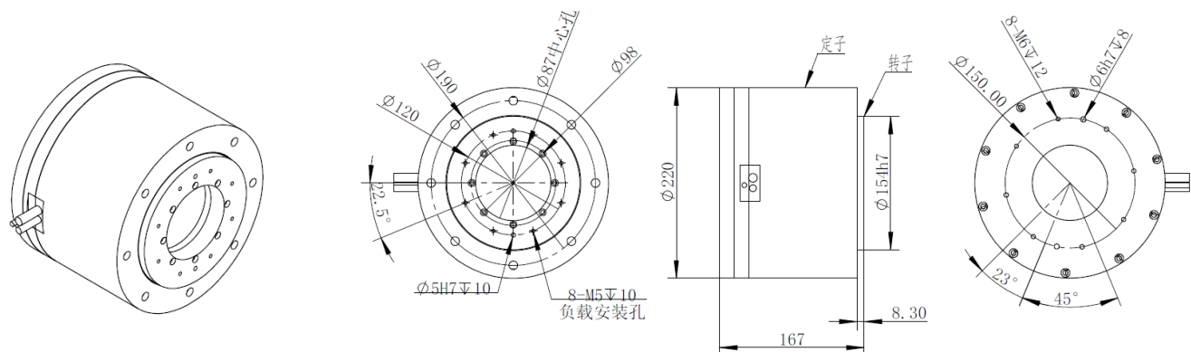
ACR220-167-H安装尺寸
