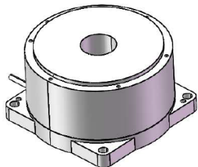
ACR170-095安装尺寸
