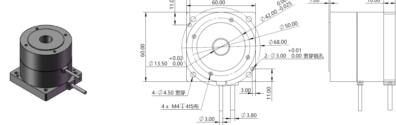
ACR60-057安装尺寸
