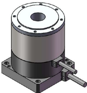
ACR40-050A安装尺寸
