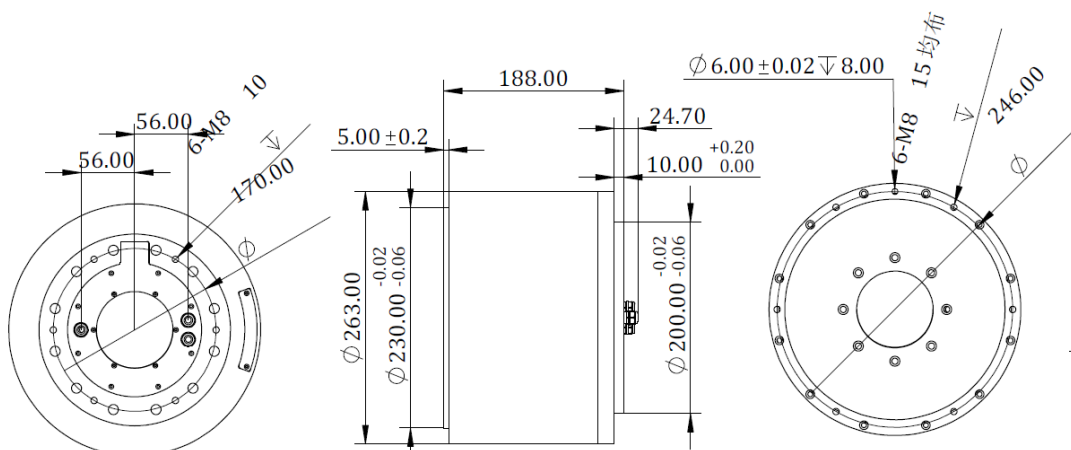
ACR263-188安装尺寸
