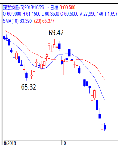
匯控(0005)日線圖
