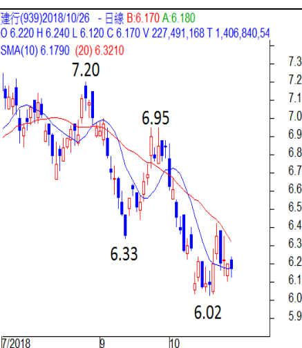
建行 (0939)日線圖
