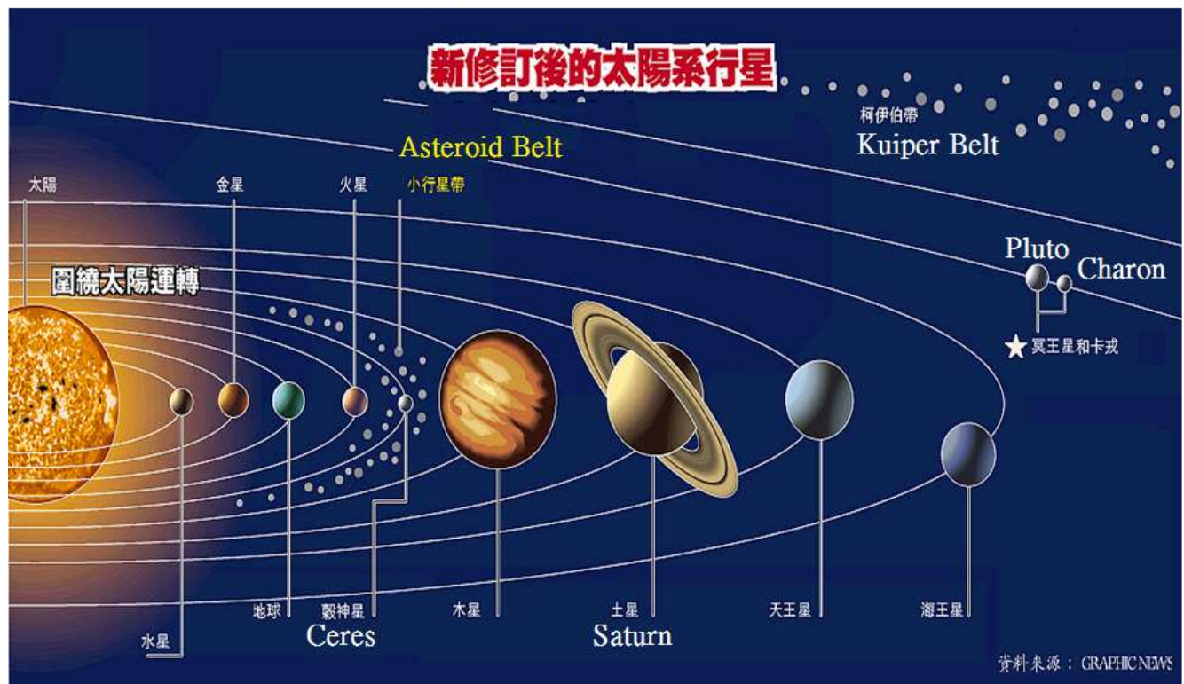
圖一：太陽系各大行星位置示意圖
