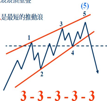
圖一：斜線三角形(diagonal triangle)示意圖
