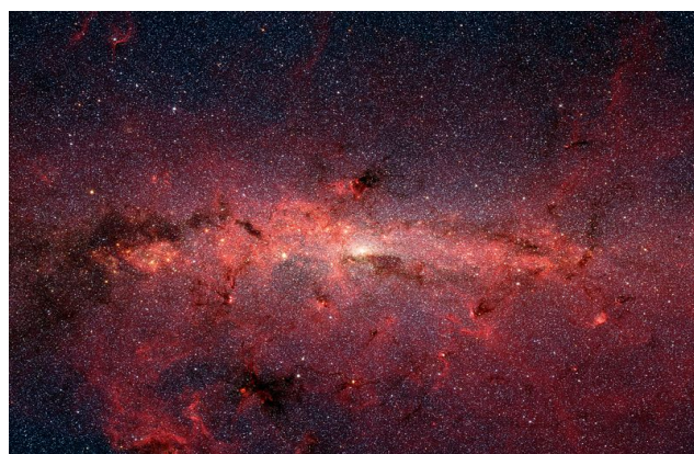
銀河中心(圖中最光的部份)
